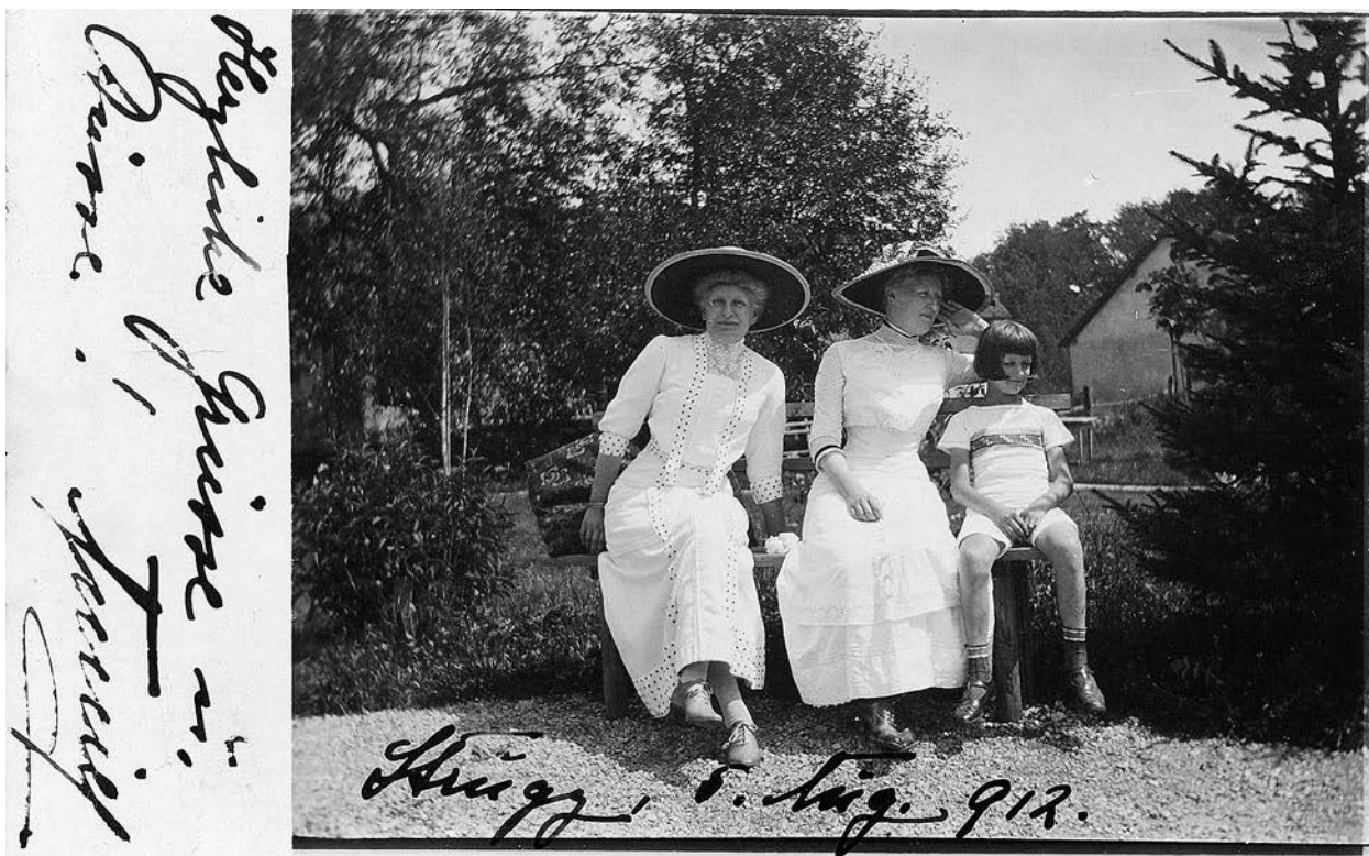
Na fotografiji so z leve proti desni: Pia pl. Fichtenau (poročena Cvitkovič), Ana Levičnik, roj. pl. Fichtenau, Toussaint (Santo) Levičnik. Struga, 1912. (Vir: SI_ZAL_NME/0182 Gospostvo Struga, t. e. 1.)
