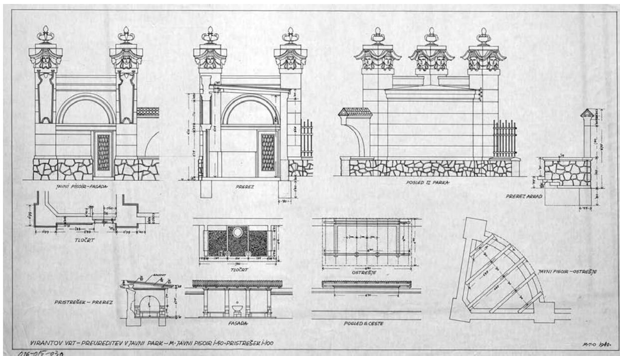
Načrt preureditve javnega parka iz leta 1942 (izris javnega pisaarja in nadstreška v vrtu) (SI ZAL LJU 334, 016-015, 30)
